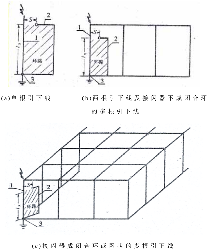
图 E.0.1 分流系数 k_c (1)
