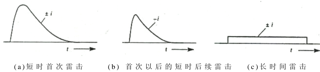
图 F.0.1-1 闪电中可能出现的三种雷击
