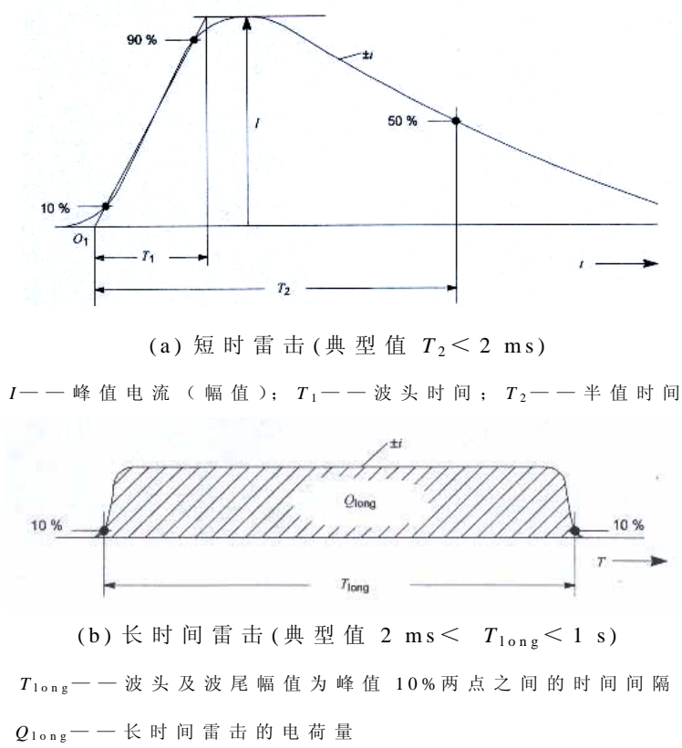
图 F.0.1-2 雷击参数定义
