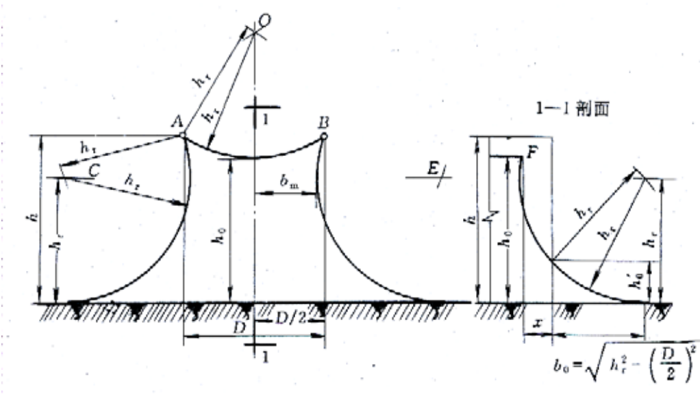
图 D.0.6-2 两根等高接闪线在高度 h 小于 2h_r 且大于 h_r 时的保护范围 1) 距地面 h_r 处作一与地面平行的线； 2) 以 A 、 B 两接闪线为圆心， h_r 为半径作弧线交于 O 点并与平行线相交或相切于 C 、 E 点； 3) 以 O 点为圆心、 h_r 为半径作弧线交于 A 、 B 点； 4) 以 C 、 E 为圆心， h_r 为半径作弧线交于 A 、 B 并与地面相切； 5) 两根接闪线之间保护范围最低点的高度 h_0 按下式计算。
