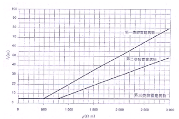
图 2 按防雷建筑物类别确定的接地体最小长度 环形接地体（或基础接地体），其所包围的面积 A 的平均几何半
