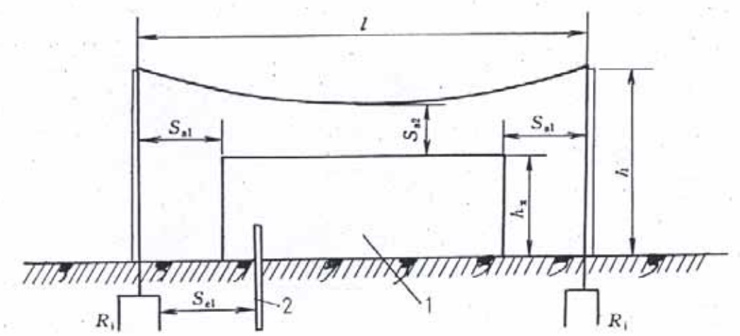
图 4.2.1 防雷装置至被保护物的间隔距离
