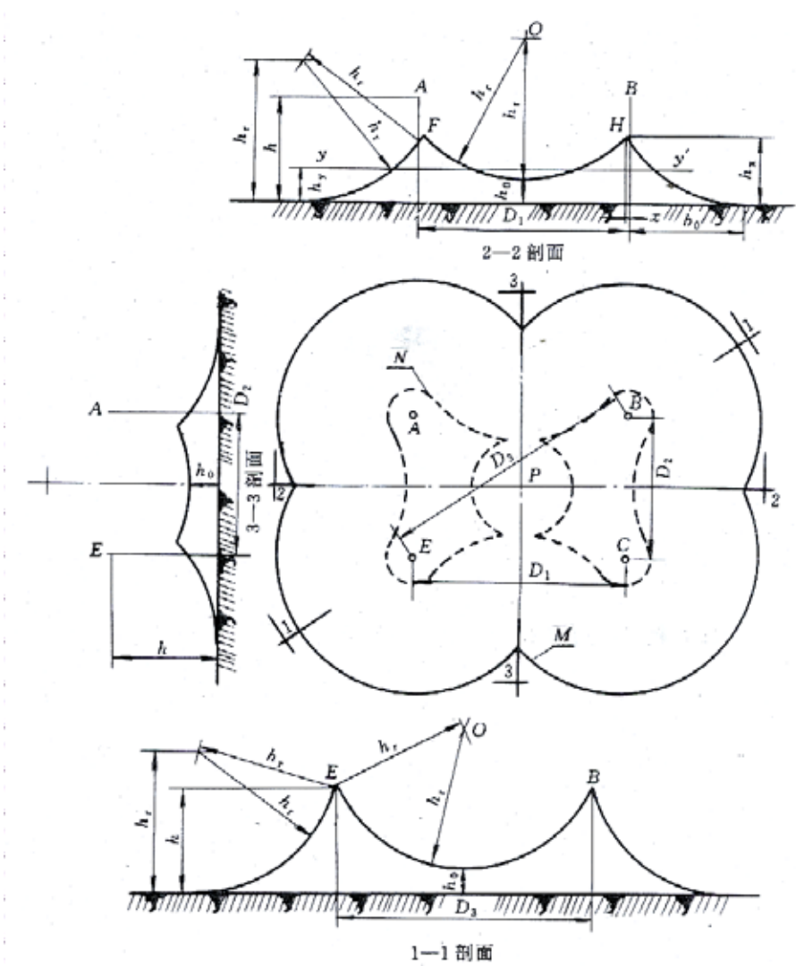
图 D.0.4 四支等高接闪杆的保护范围
