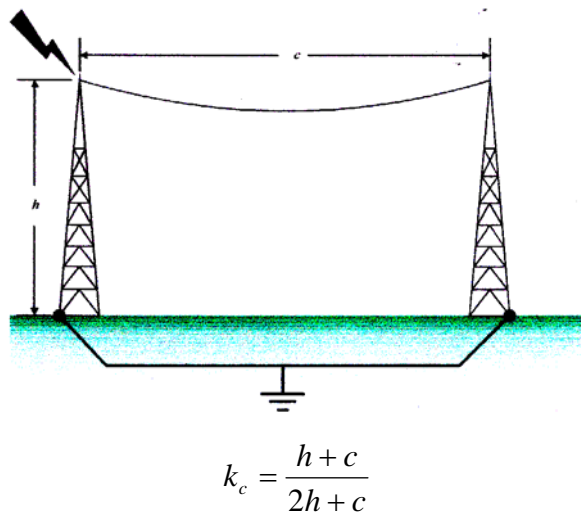
图 E.0.4 分流系数 k_c (3)
