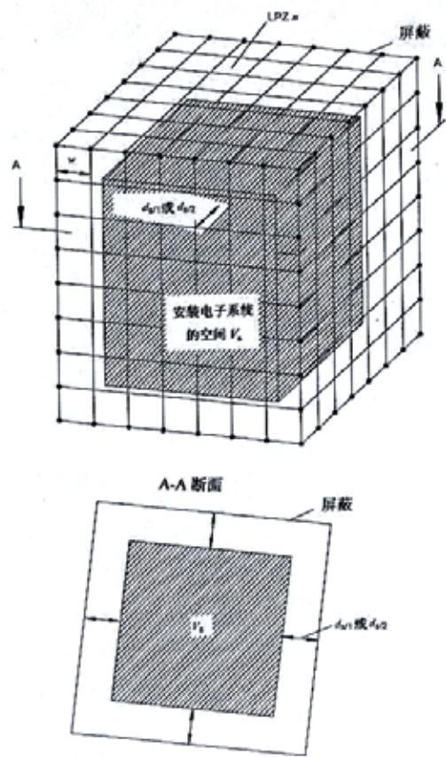
图 6.3.2-3 在 LPZ n 区内供安放电气和电子系统的空间 注：空间 V_s 为安全空间。
