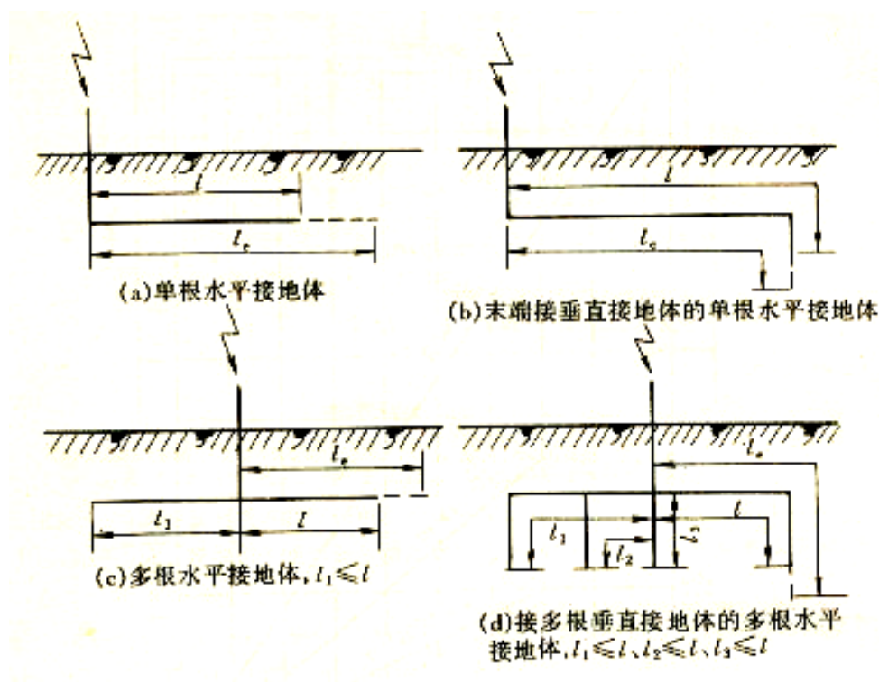
图 C.0.2 接地体有效长度的计量
