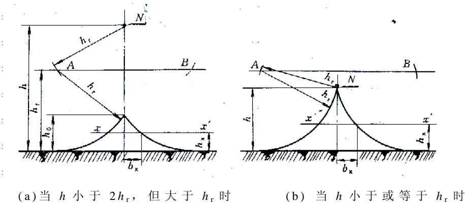
图 D.0.5 单根架空接闪线的保护范围
