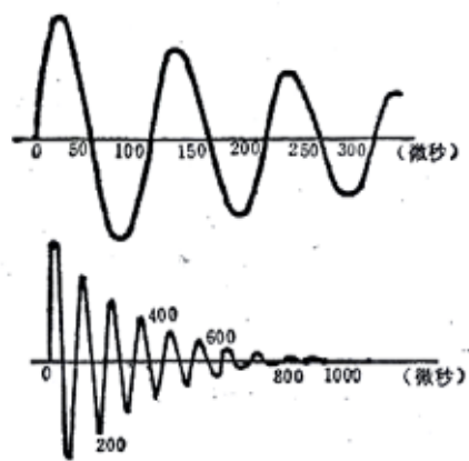
图 10 具有代表性的冲击电流波形
