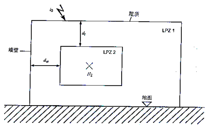
图 6.3.2-5 LPZ 2 区内的磁场强度
